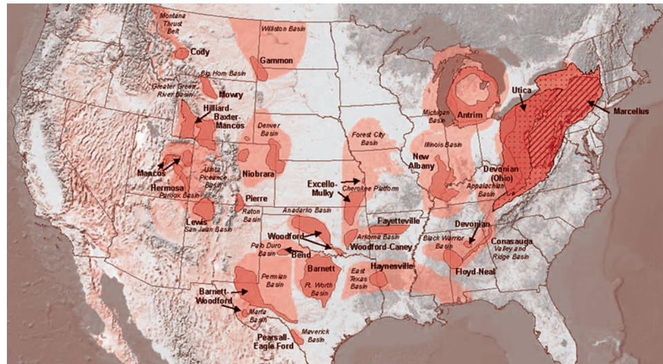
Залежи сланцевого газа в США, по данным Агентства энергетической информации (EIA)
