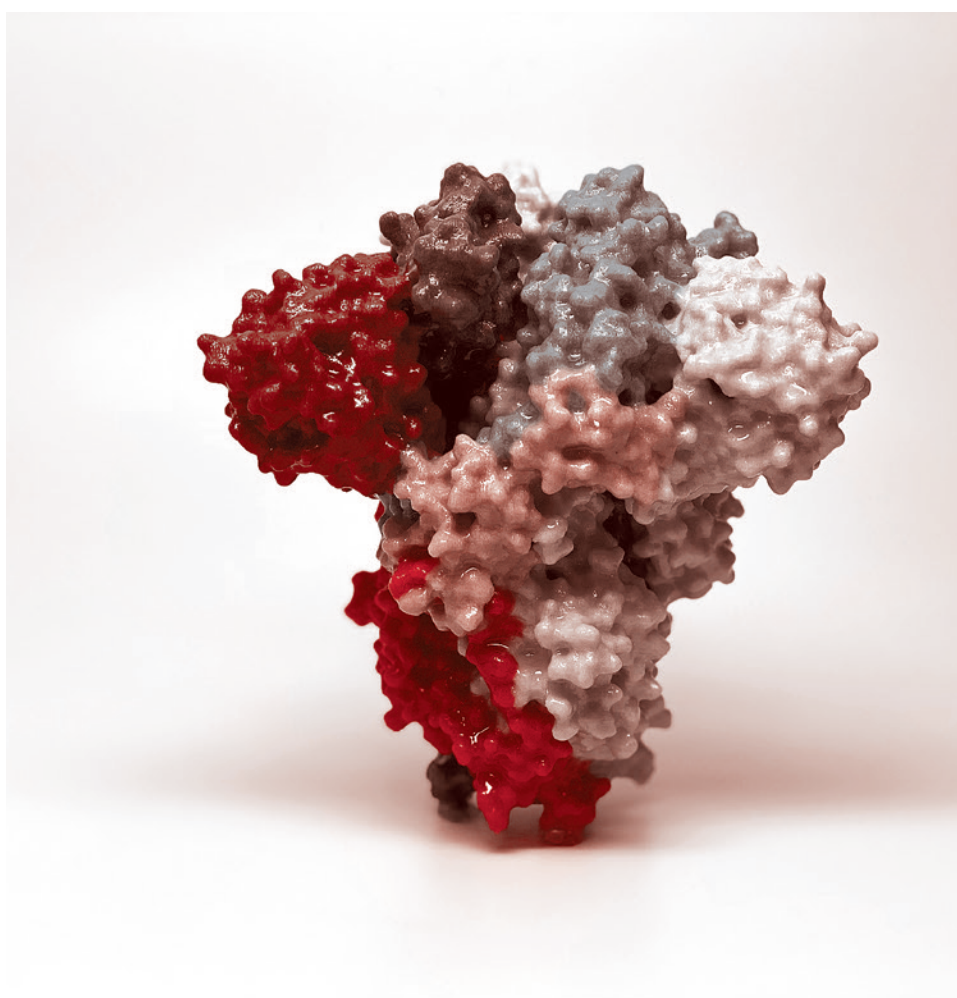
S-белок SARS-CoV-2 (3d модель NIAID)
