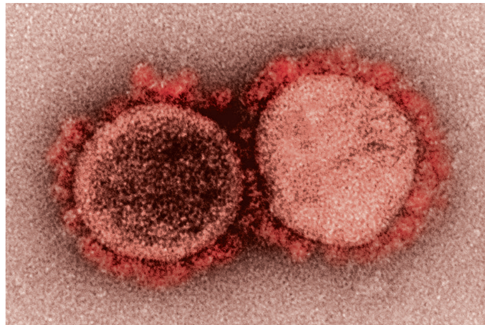
Изображение SARS-CoV-2, полученное с помощью просвечивающей электронной микроскопии в Национальном институте аллергии и инфекционных заболеваний в Форте Детрик
