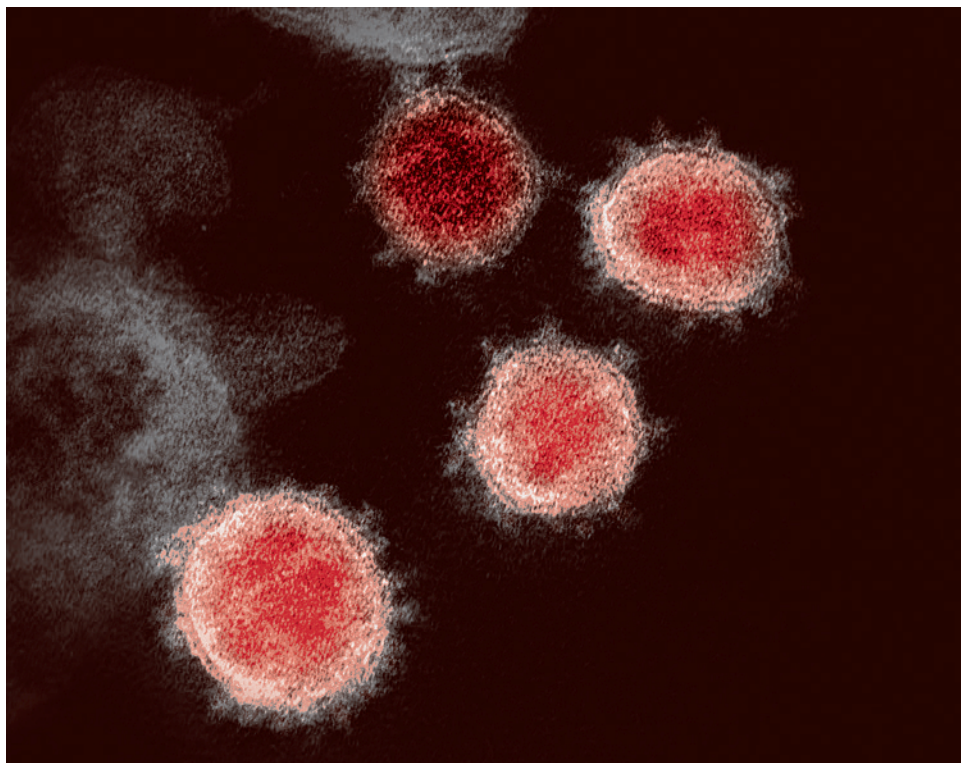
Вирус SARS-CoV-2 через просвечивающий электронный микроскоп
