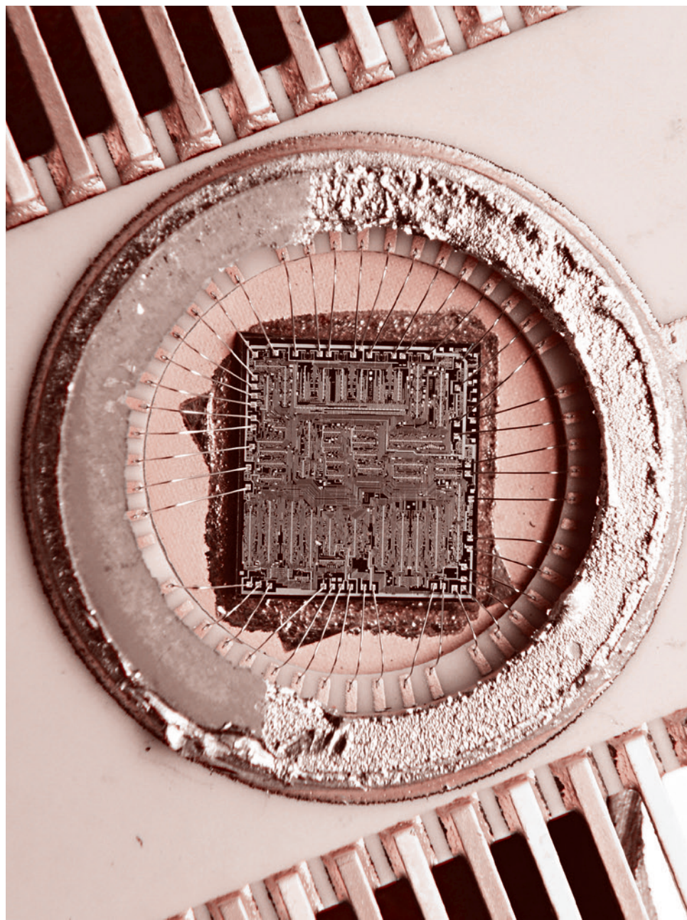
Отечественная микросхема 582ИК1 (аналог американской SBP0400) на основе которой в 1980-е годы была реализована БЦВМ «Бисер-4» системы управления орбитального корабля «Буран»
