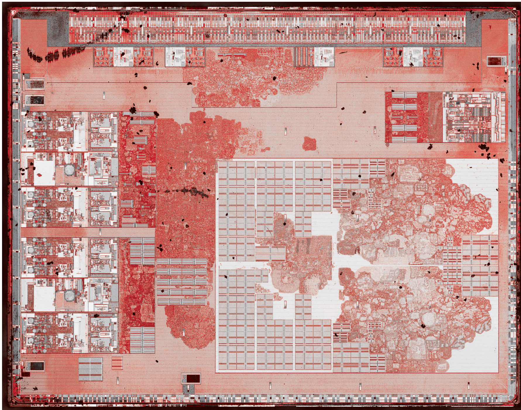
Процессор Baikal-T1 после снятия металлизации (фото — BarsMonster, habr.com)
