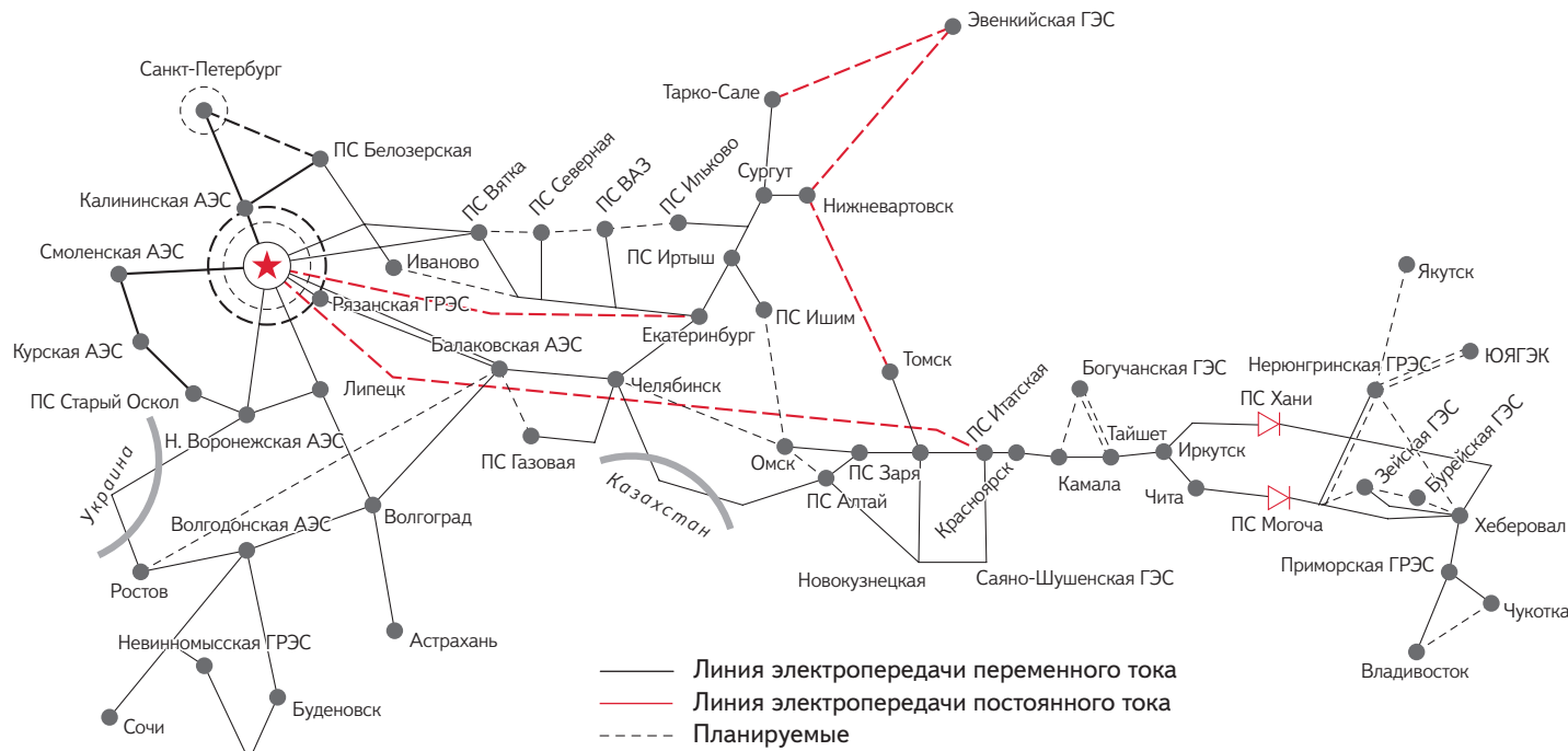
Рис. 4. Схема развития основной электрической сети Российской Федерации
