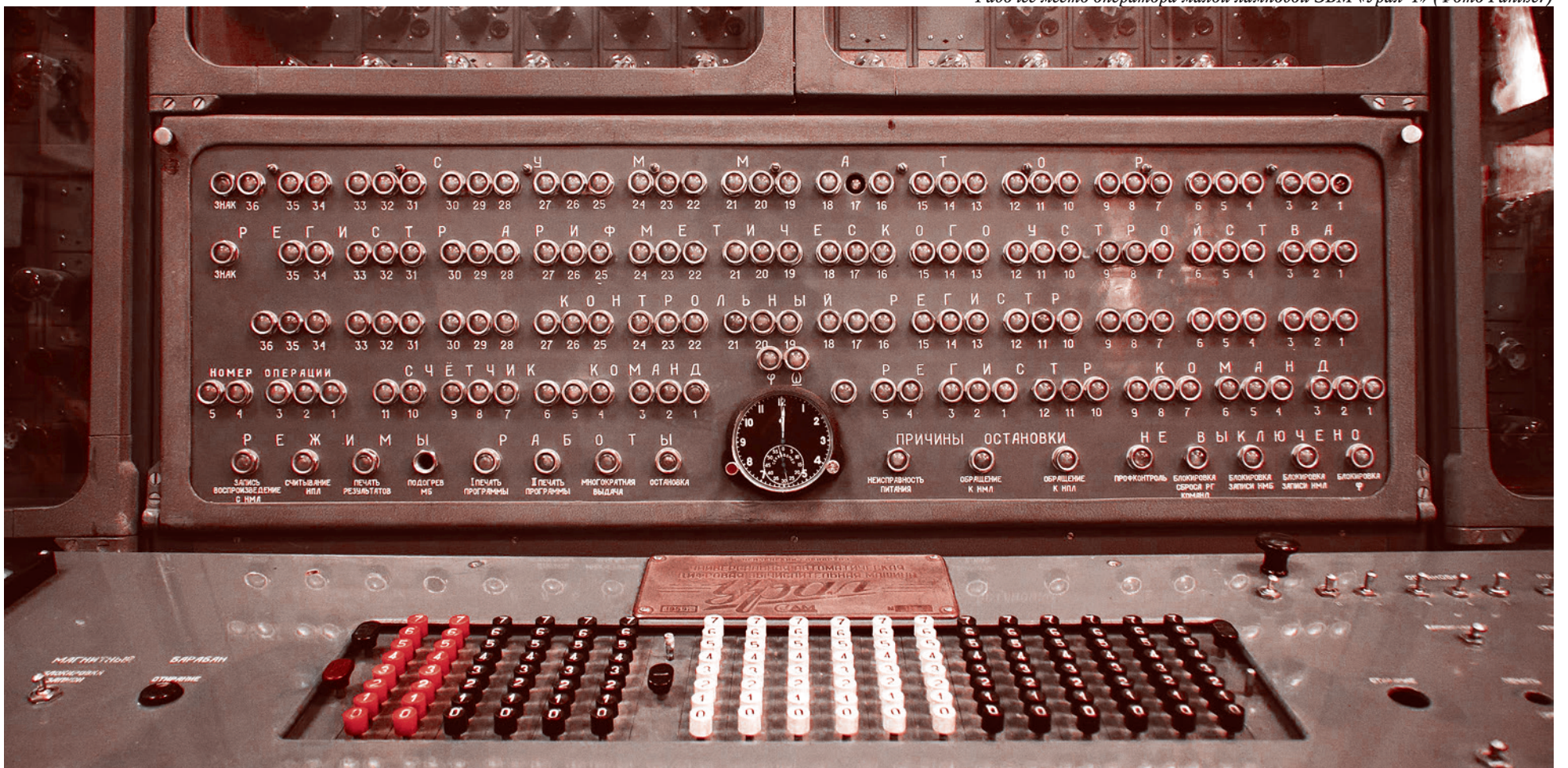
Рабочее место оператора малой ламповой ЭВМ «Урал-1» (Фото Panther)
