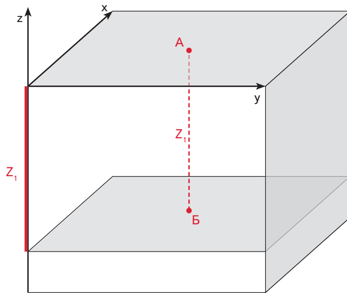
Рис. 6. Трехмерное пространство
